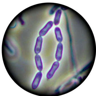
Metarhizium anisopliae
